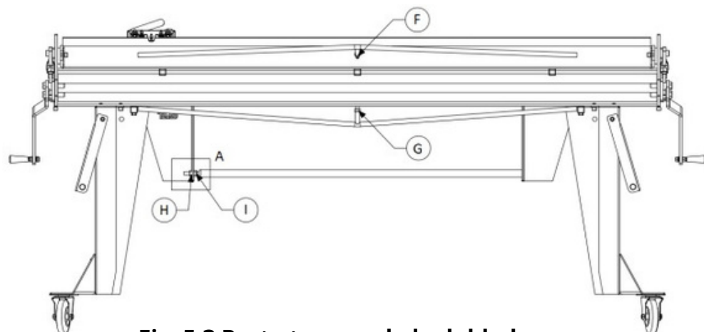
Fig. 5.3 Parte trasera de la dobladora
