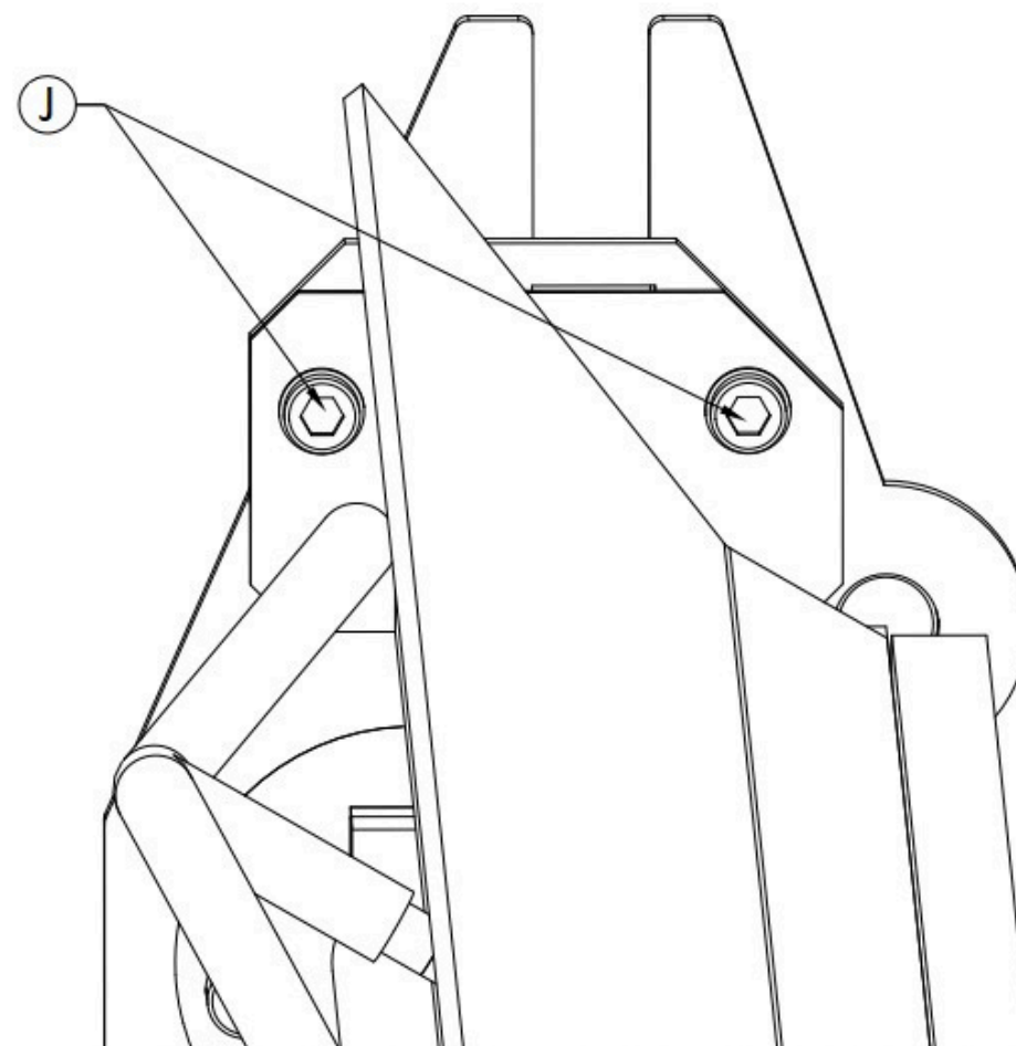
Fig. 5.5 Fijación de la viga de sujeción superior
