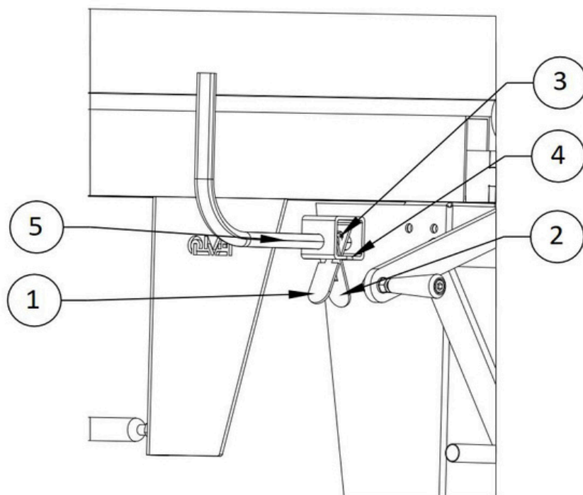
Fig. 5.6 Mecanismo de bloqueo del parachoques
