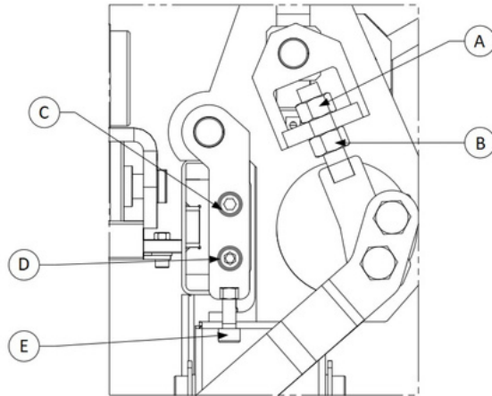
Fig. 5.1 Lado de la máquina dobladora
